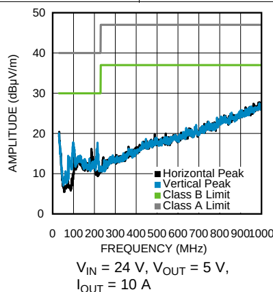
Figure 52. Radiated EMI (EN 55022)
