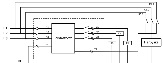
Рис.1б. Управление нагрузкой через магнитные пускатели (&gt;8А)
