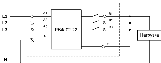
Рис. 1а. Прямое подключение к нагрузке (&lt;8А)
